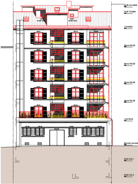
Coupes façade sud-ouest Schnitte Südwestfassade
