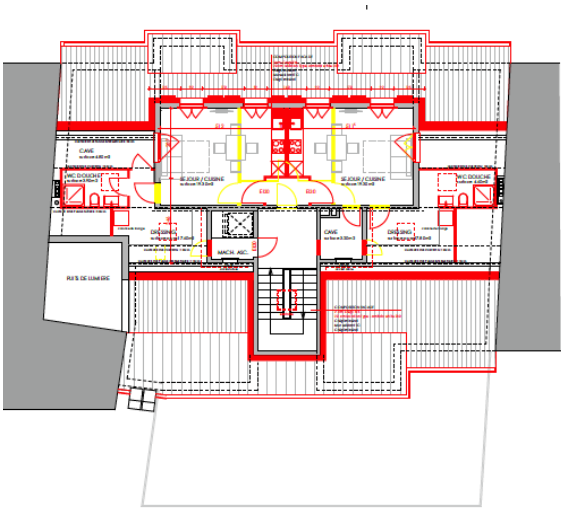
Plan des combles Dachbodenplan
