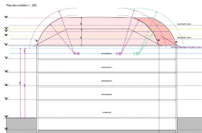
Coupe façades Schnitt Fassaden
